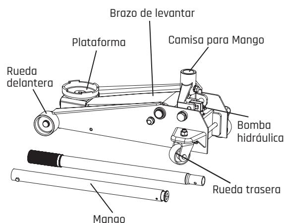
FIGURA1 - GATO DE SERVICIO
